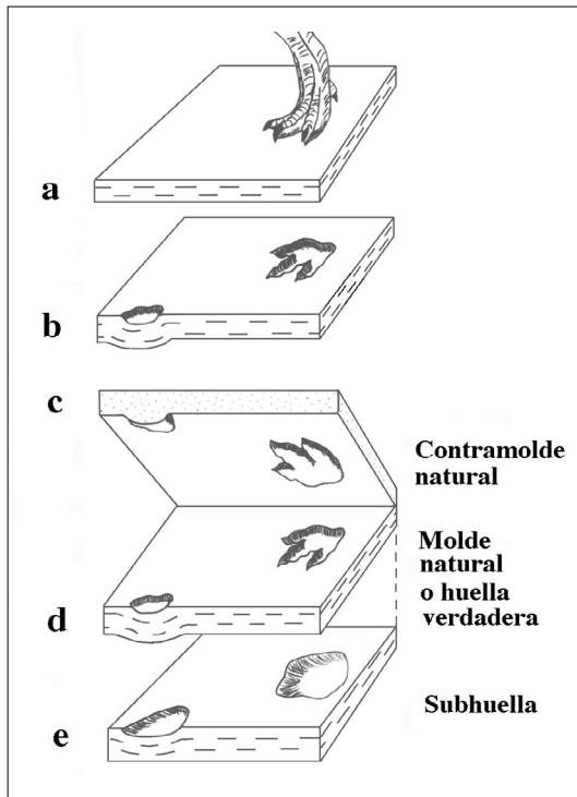
Fig. 2. Esquema de formación de una huella (a y b). Distintos tipos de conservación de icnitas en el registro geológico (c, d y e).
