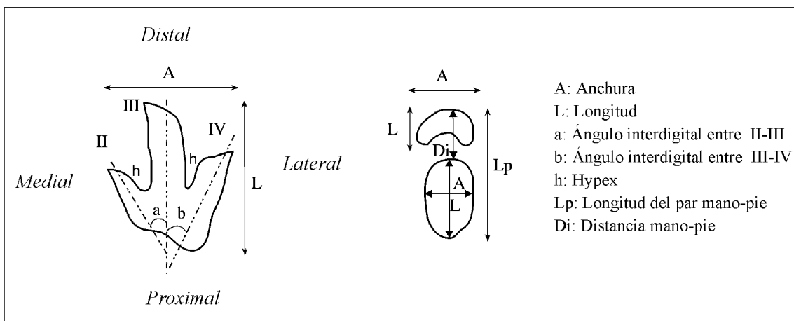
Fig. 3. Medidas a realizar en icnitas individuales de dinosaurios bípedos (izquierda) y cuadrúpedos (derecha).
