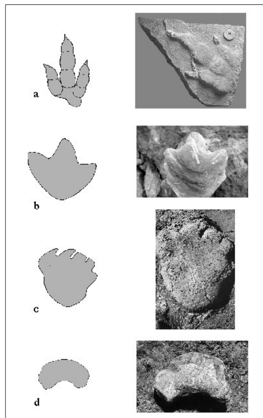
Fig. 1. Morfología de las huellas de los tres grupos principales de dinosaurios: (a) terópodo, (b) ornitópodo, (c y d) pie y mano de saurópodo respectivamente.
