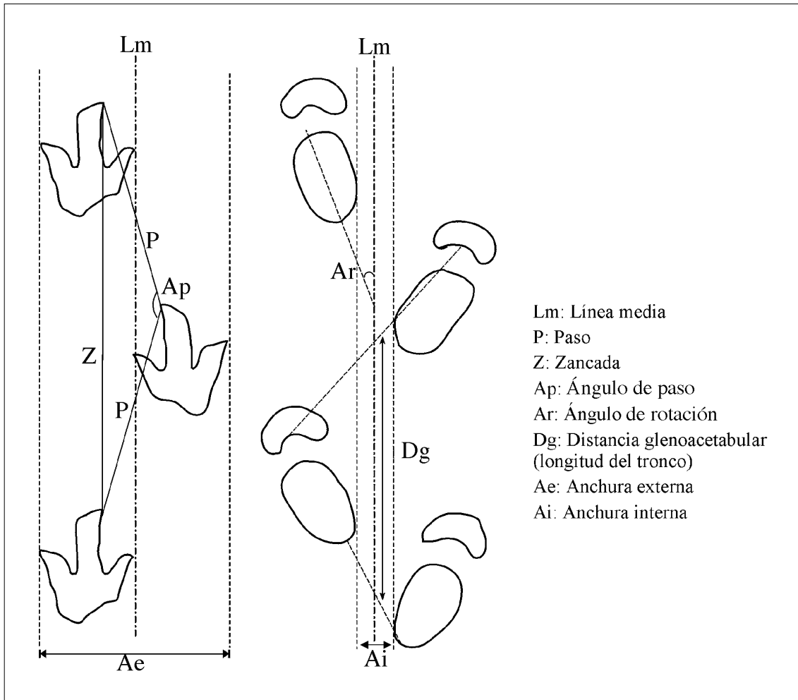
Fig. 4. Medidas a realizar en rastros de dinosaurios bípedos (izquierda) y cuadrúpedos (derecha).
